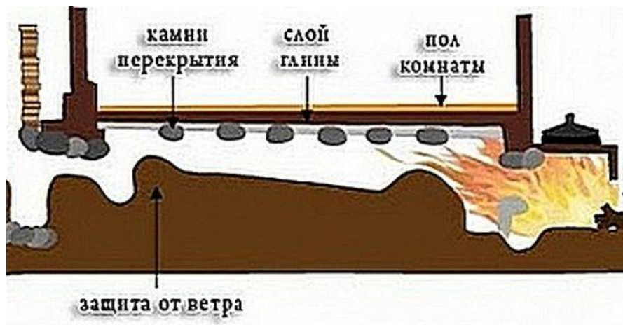
Кан. Система отопления.
